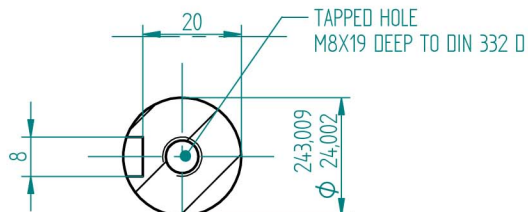
Przekrój A-A 1:1
